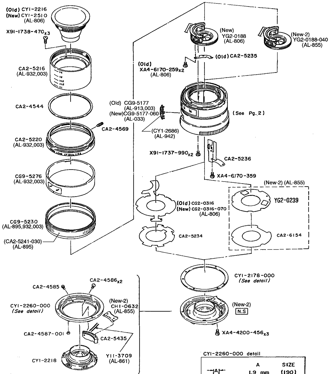
CY1-2178-000 detail
