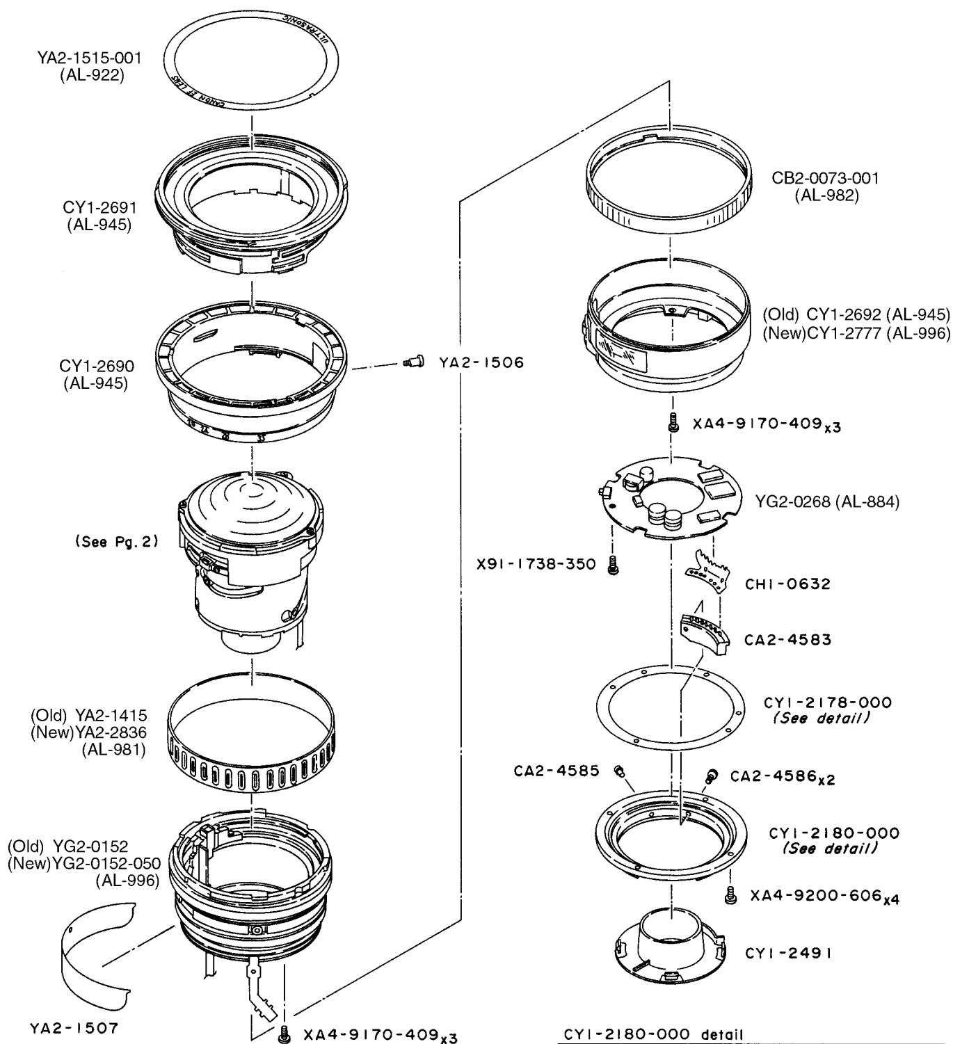
CY1-2178-000 detail
