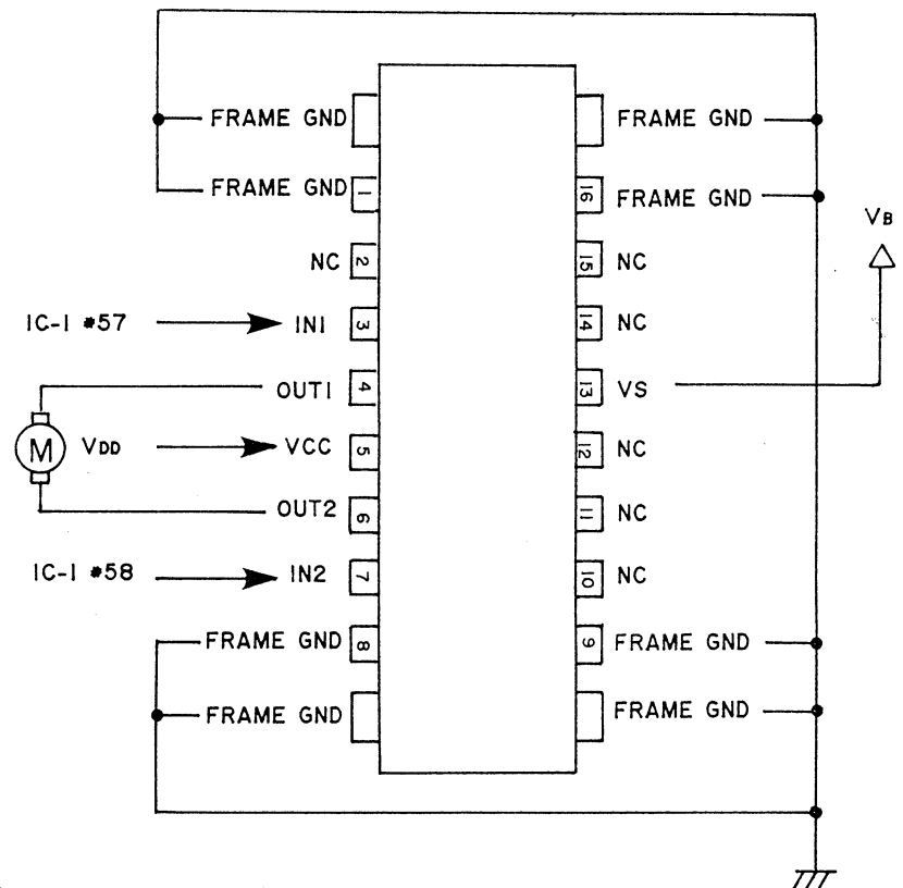
AF Drive IC (IC-6)
