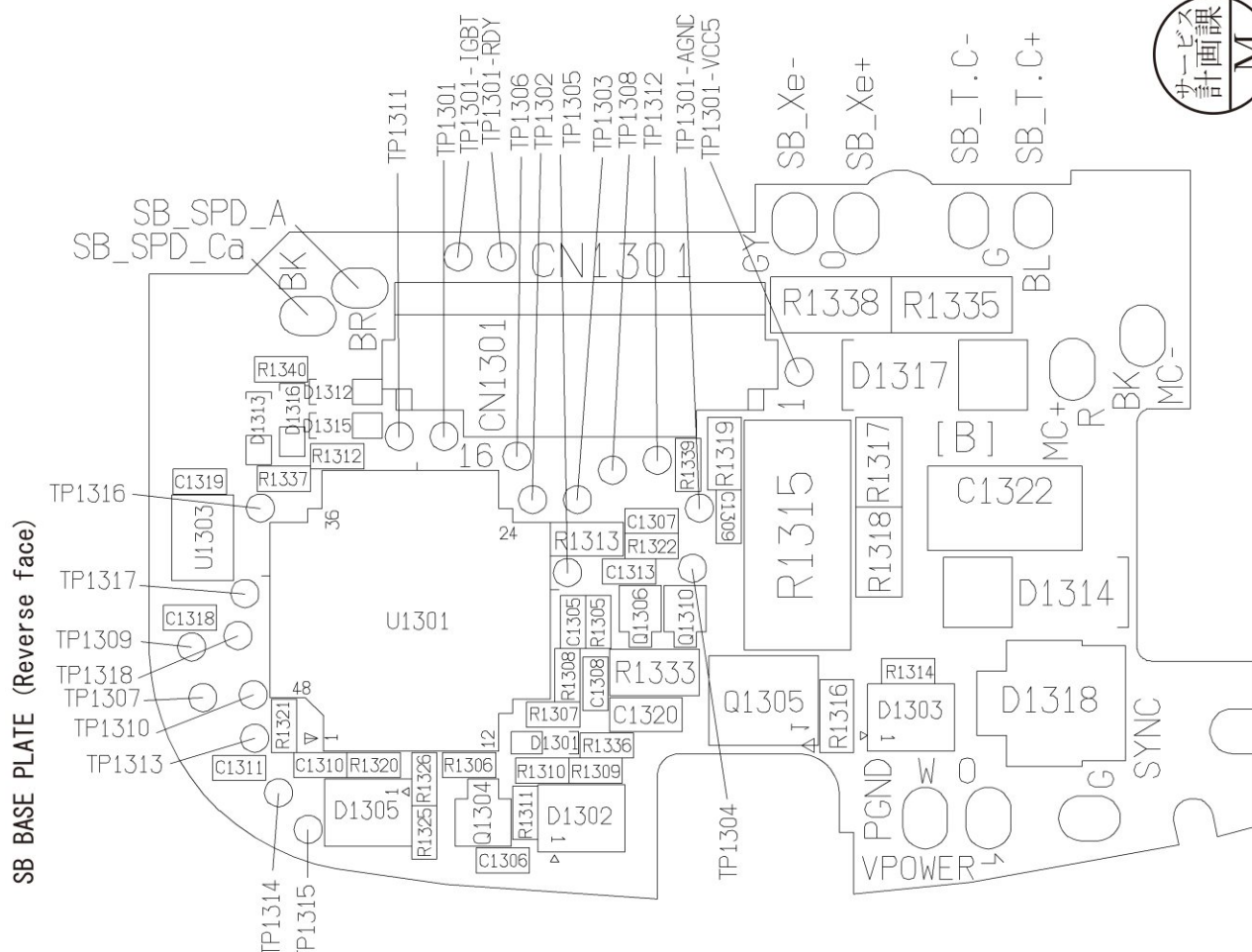
SB 基板 (裏)
