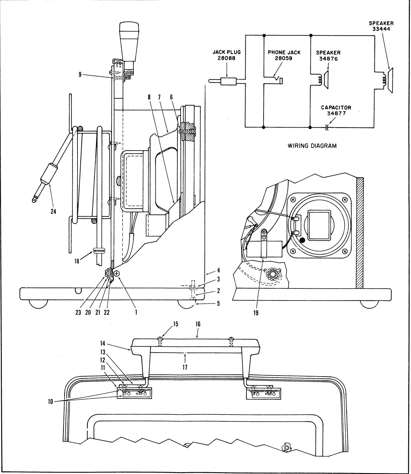
Figure 37. Dual AV Speaker Assembly
