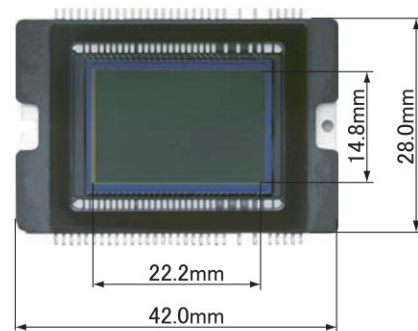
Fig. 001 CMOS sensor
