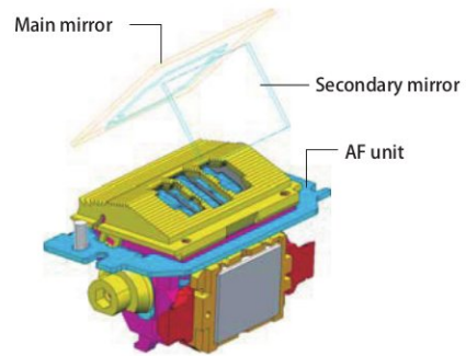
Fig. 012 AF unit
