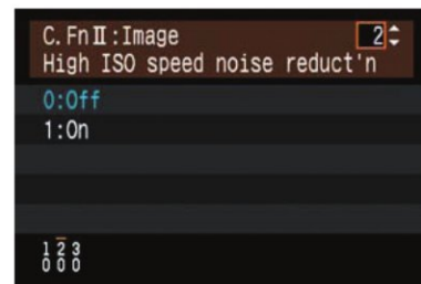
Fig. 006 C.Fn II-2
