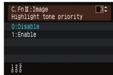
Fig. 007 C.Fn II-3
