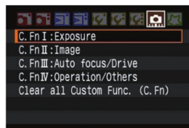
Fig. 024 Custom Functions
