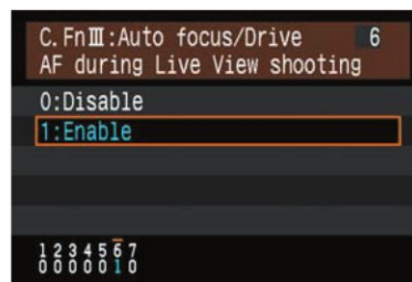
Fig. 022 C.Fn-III-6
