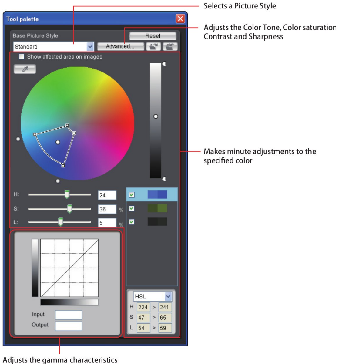
Fig. 007 Tool palette
