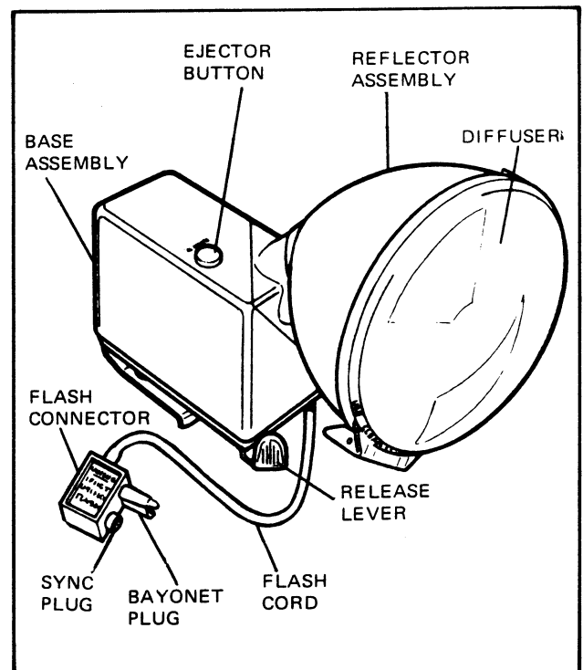
FIG. 2.15 FLASHGUN
