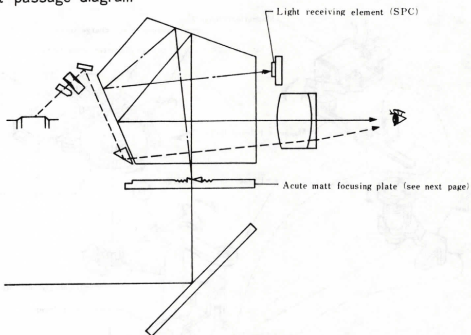
7-1. Light passage diagram
