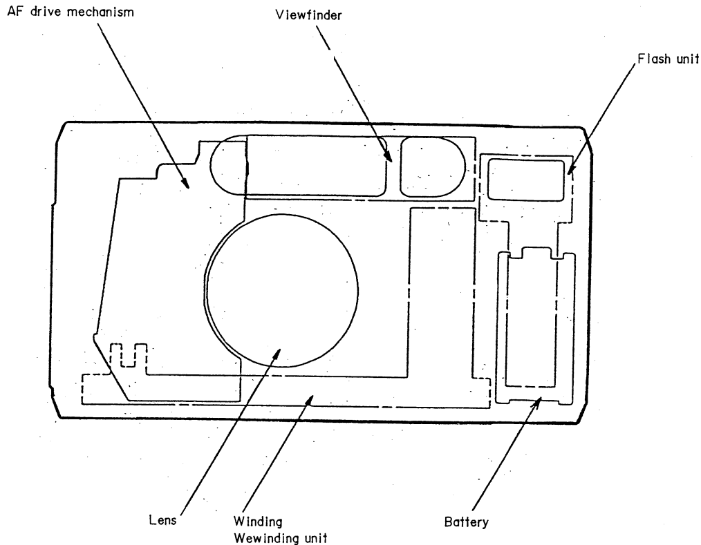
[Unit Layout]
