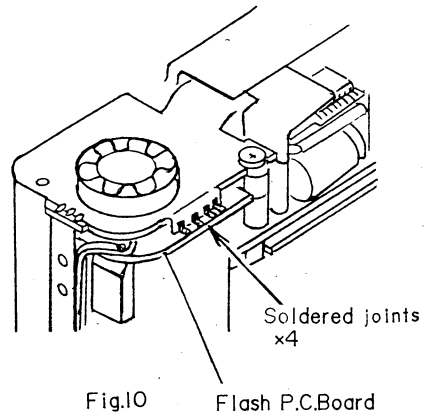
Fig.10 Flash P.C.Board
